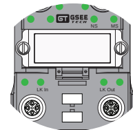
EtherCAT Net_In/Out 通讯口
