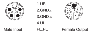
M12 L-CODE接插件电源供电, U B 为系统电源, U L 为负载电源
