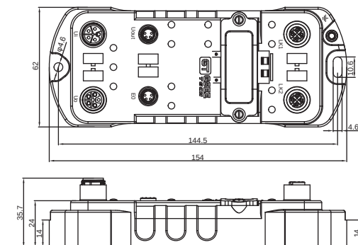
模块外形规格
