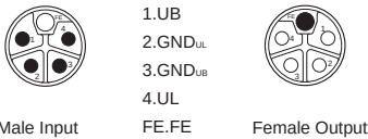
M12 L-CODE接插件电源供电, U B 为系统电源, U L 为负载电源
