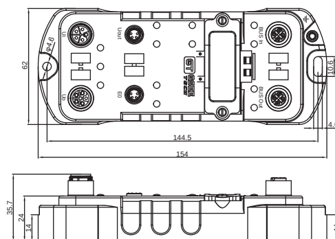
模块外形规格
