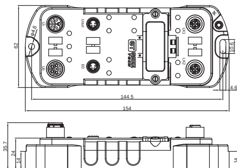
模块外形规格
