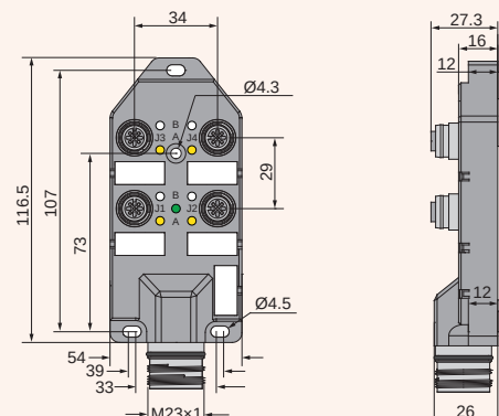
外形尺寸 接线图
