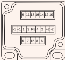
接线盒 21-Pin
