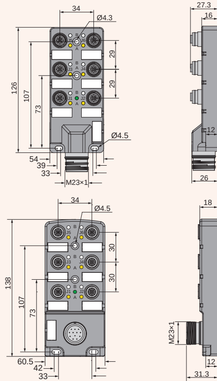
外形尺寸 接线图
