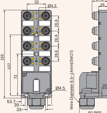
外形尺寸 接线图
