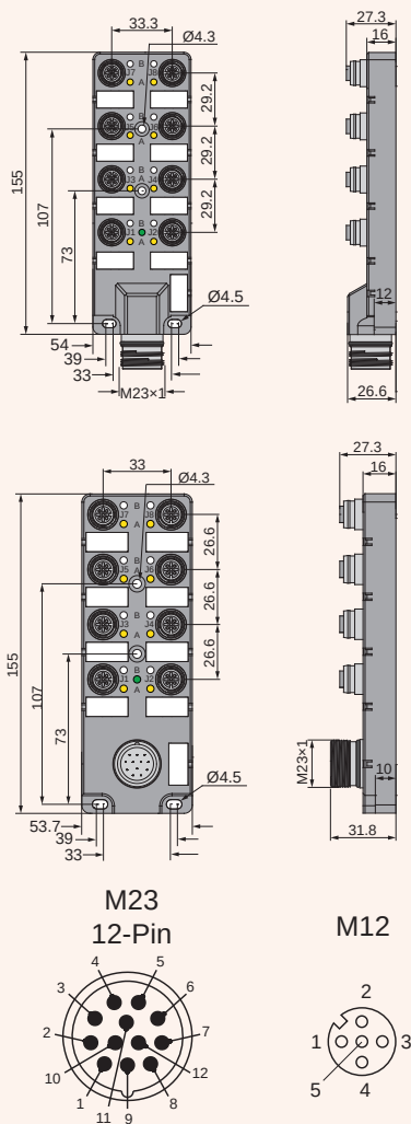
外形尺寸 接线图
