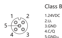
M12 A-Code IO-Link 端口接线示意
