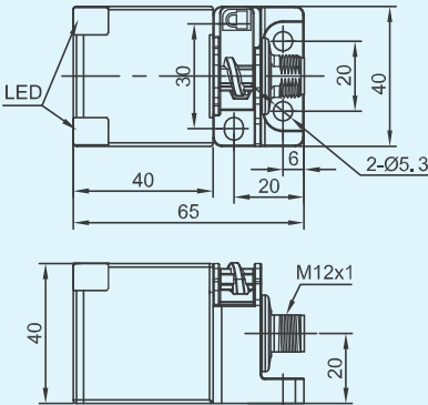
标准电感式传感器，P40 标准方形外壳，DC 3 /4线，供电电压：10...30 VDC
