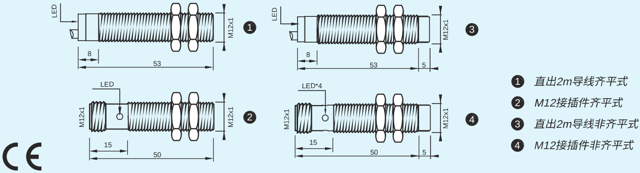
低温型电感式传感器，M12圆柱螺纹型外壳，DC 2线3线（10...30 VDC）或交流两线 20...250 VAC
